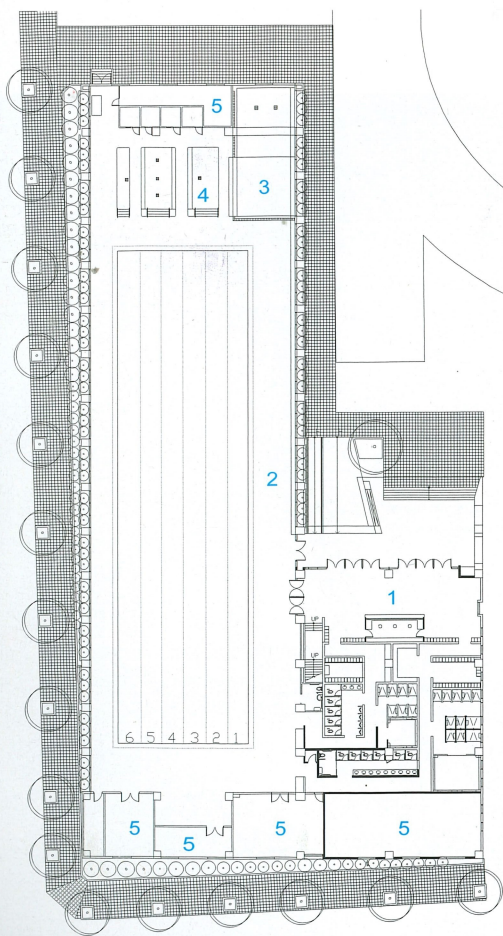
游泳館一層平面圖
