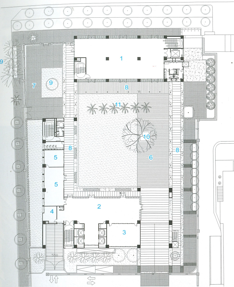
美術館、綜合教學大樓一層平面圖
